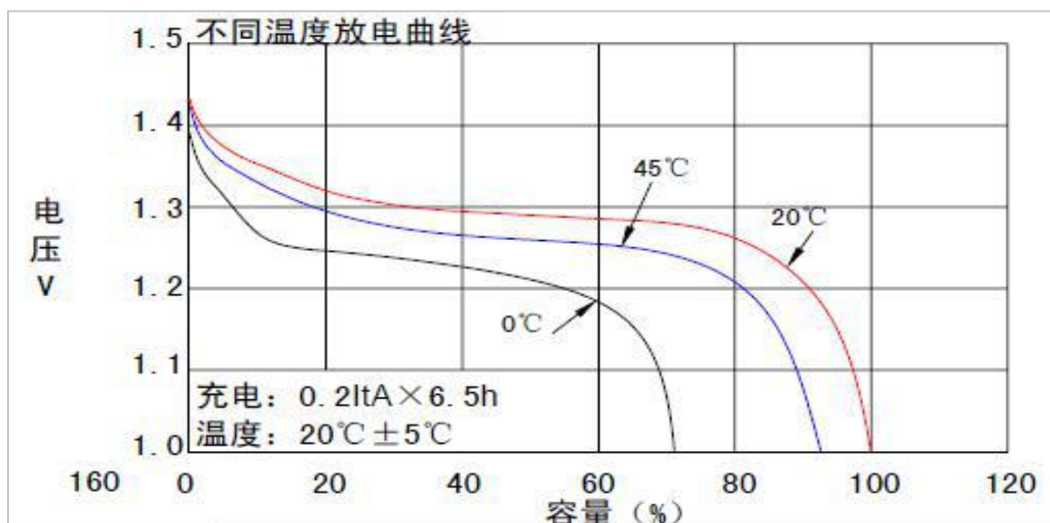
特征曲线
